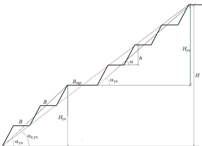
Рисунок 1. Схема конструкции бортов и уступов: h , H_{уч} , H – соответственно высота уступа, групп уступов, борта; \alpha_y , \alpha_{к.уч} , \alpha – соответственно, угол откоса уступа, конструктивной группы уступов и борта карьера, разреза; B , B_{mp} – соответственно, ширина предохранительной и транспортной бермы
