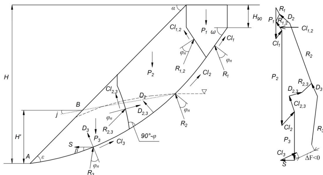
Рисунок 3 – Схема расчета устойчивости обводненного изотропного откоса с учетом воздействия сейсмических сил методом векторного сложения сил: P_i – вес рассматриваемого блока, мН; Cl_{i,i+1} , Cl_{i,i-1} , Cl_i – силы сцепления, направленные параллельно соответствующим границам блоков, мН; D_{i,i+1} , D_{i,i-1} , D_i – силы гидростатического давления по границам блоков, мН; R_{i,i+1} , R_{i,i-1} , R_i – реакции по границам блоков, мН; S – сейсмическая сила, мН; \beta – угол наклона сейсмической силы, град.
