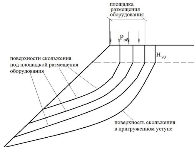
Рисунок 4 – Схема расчета устойчивости уступа с учетом влияния веса оборудования, зданий, сооружений
